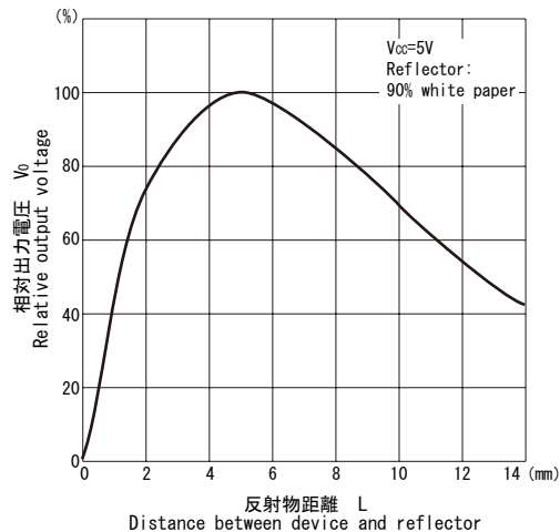
■ 相対出力電圧/距離特性 V_o/L
